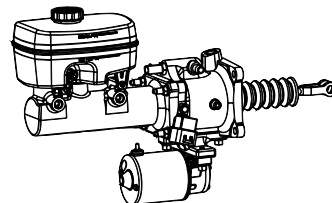
Illustration 44 : Ensemble servofrein et maître-cylindre
