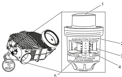
Illustration 24 : Indicateur de colmatage du filtre à air
