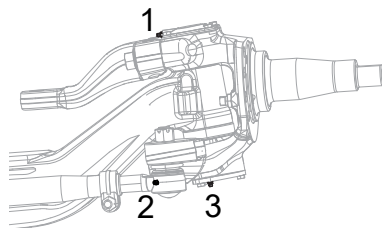
Illustration 49 : Points de graissage pour essieu avant FX-20 PACCAR
