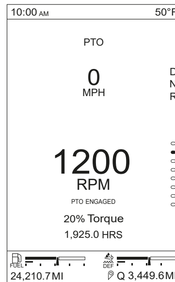
Illustration 11 : Prise de force électronique (PDF) engagée
