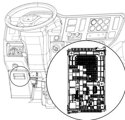
Illustration 7 : Accès au porte-fusibles
