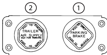
Illustration 27 : Combinaison (véhicule/remorque) des soupapes de commande des freins de stationnement
