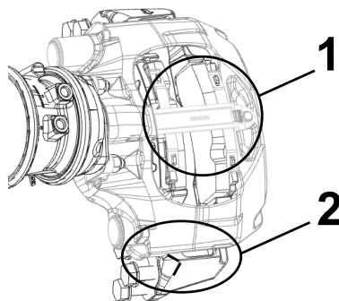
Illustration 42 : Détails de l'étrier
