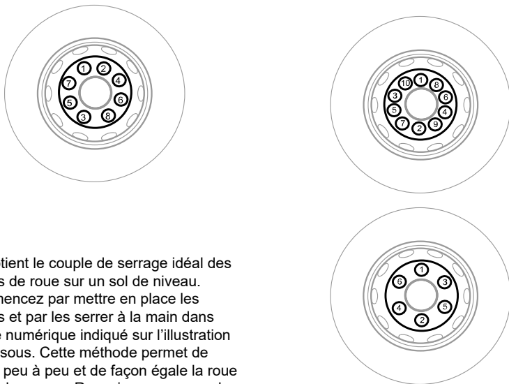
Illustration 52 : Roues à disque centrées par goujons
