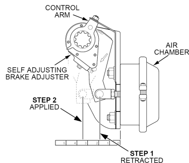
Illustration 43 : Course de l'actionneur de freins
