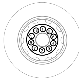
Illustration 51 : Roues à disque centrées par moyeu
