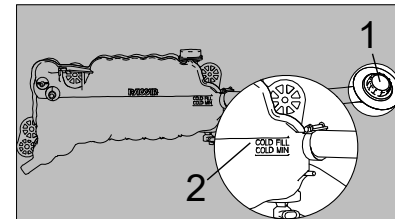
Illustration 46 : Réservoir d'équilibre de liquide de refroidissement monté sur cloison
