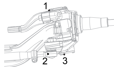
Illustration 49 : Points de graissage pour essieu avant 20 000 PACCAR
