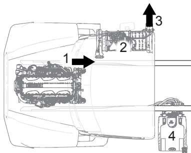
Illustration 36 : Épure du système de post-traitement du moteur
