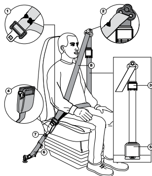
Illustration 46 : Points de contrôle des ceintures de sécurité
