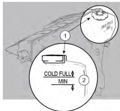
Illustration 45 : Réservoir de surtension de liquide de refroidissement monté sur radiateur
