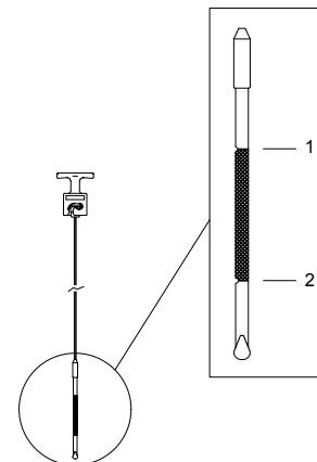
Illustration 48 : Repères de la jauge d'huile à moteur
